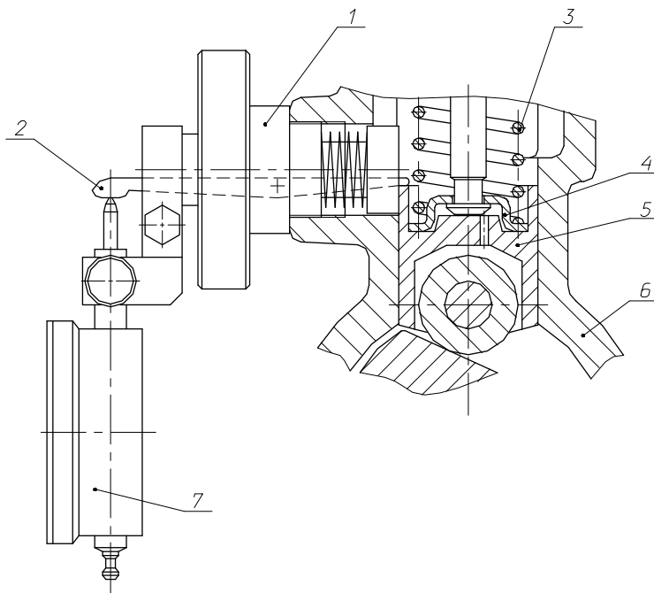
Рис. 15. Измерение величины подъема толкателя:
